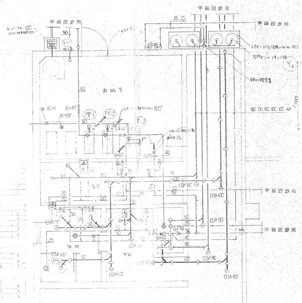
1階トイレ室平面図詳細図 1/50
