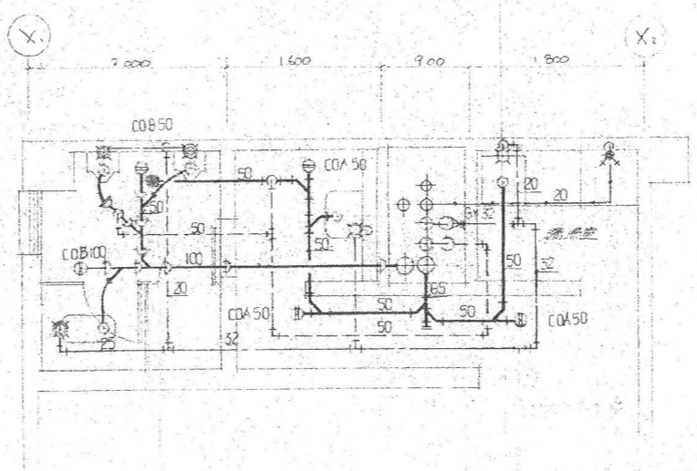
2階トイレ洗面場詳細図 1/50
