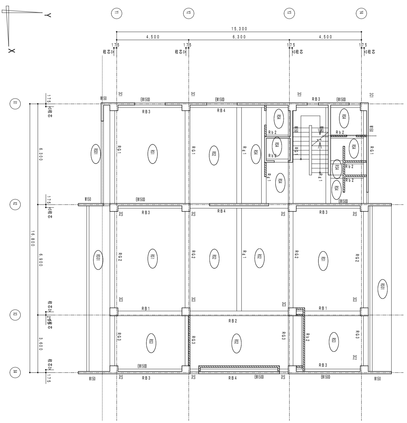
2階梁伏図 1/100
