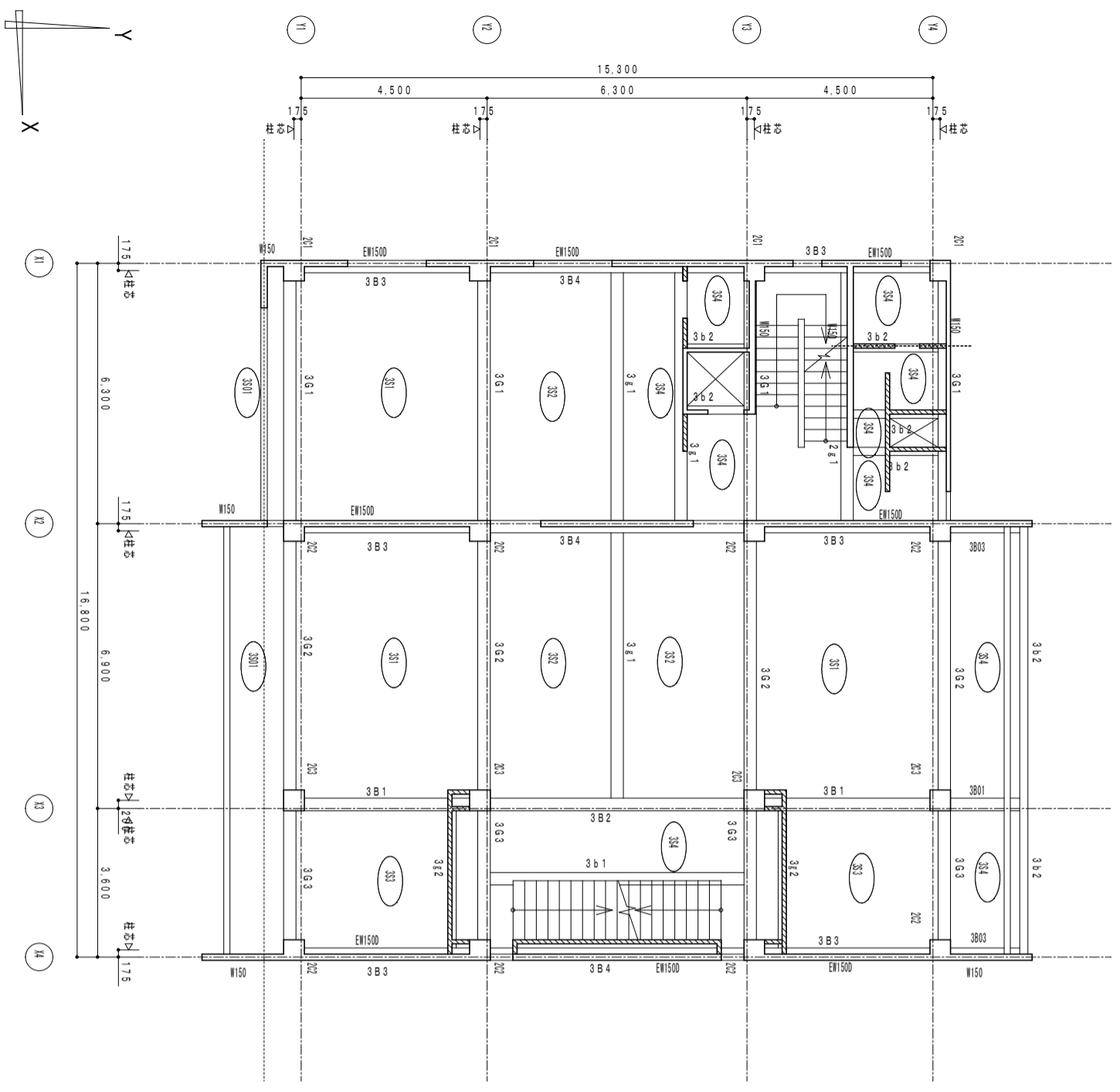
3階梁伏図 1/100
