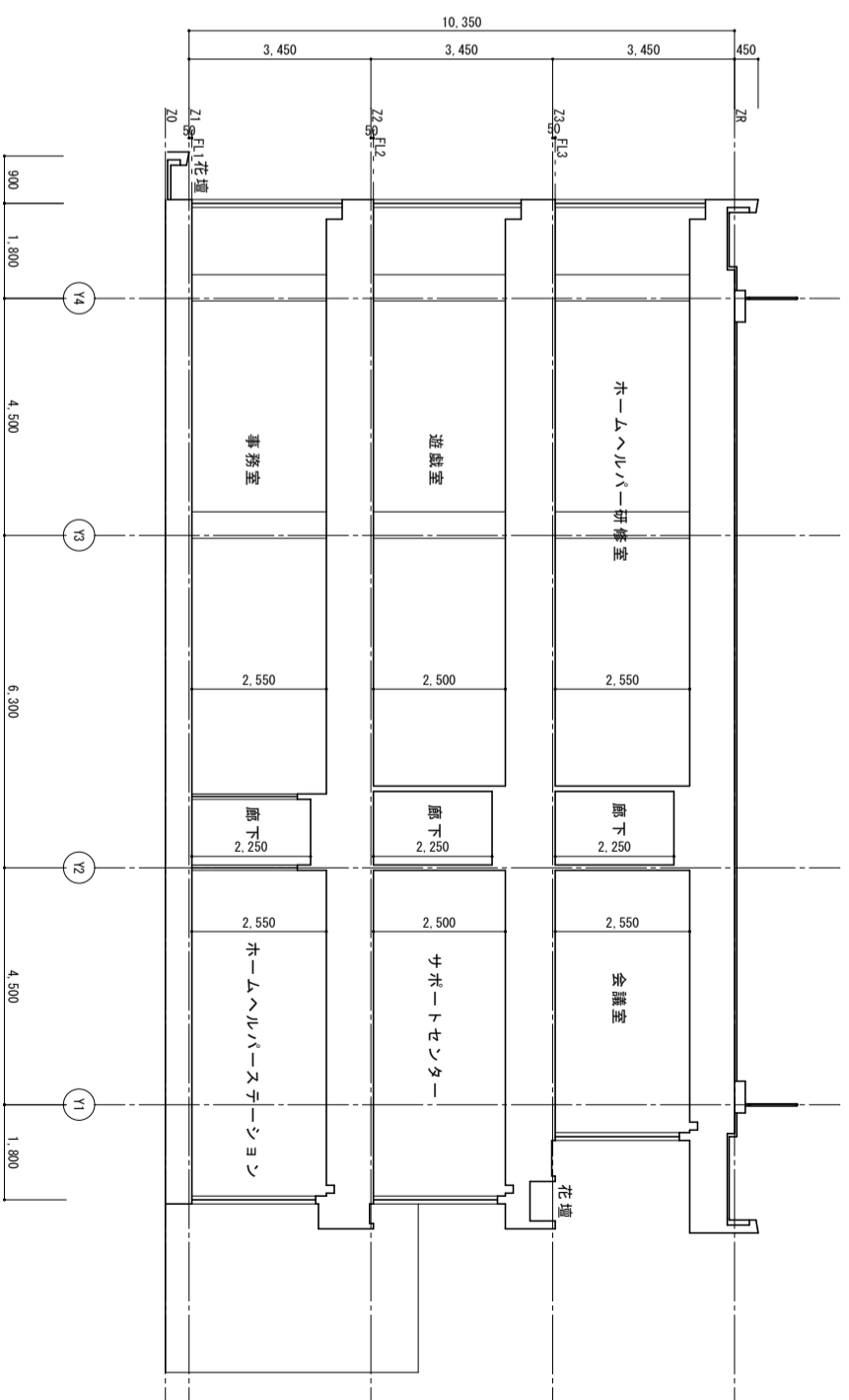
Y-Y' 断面図
