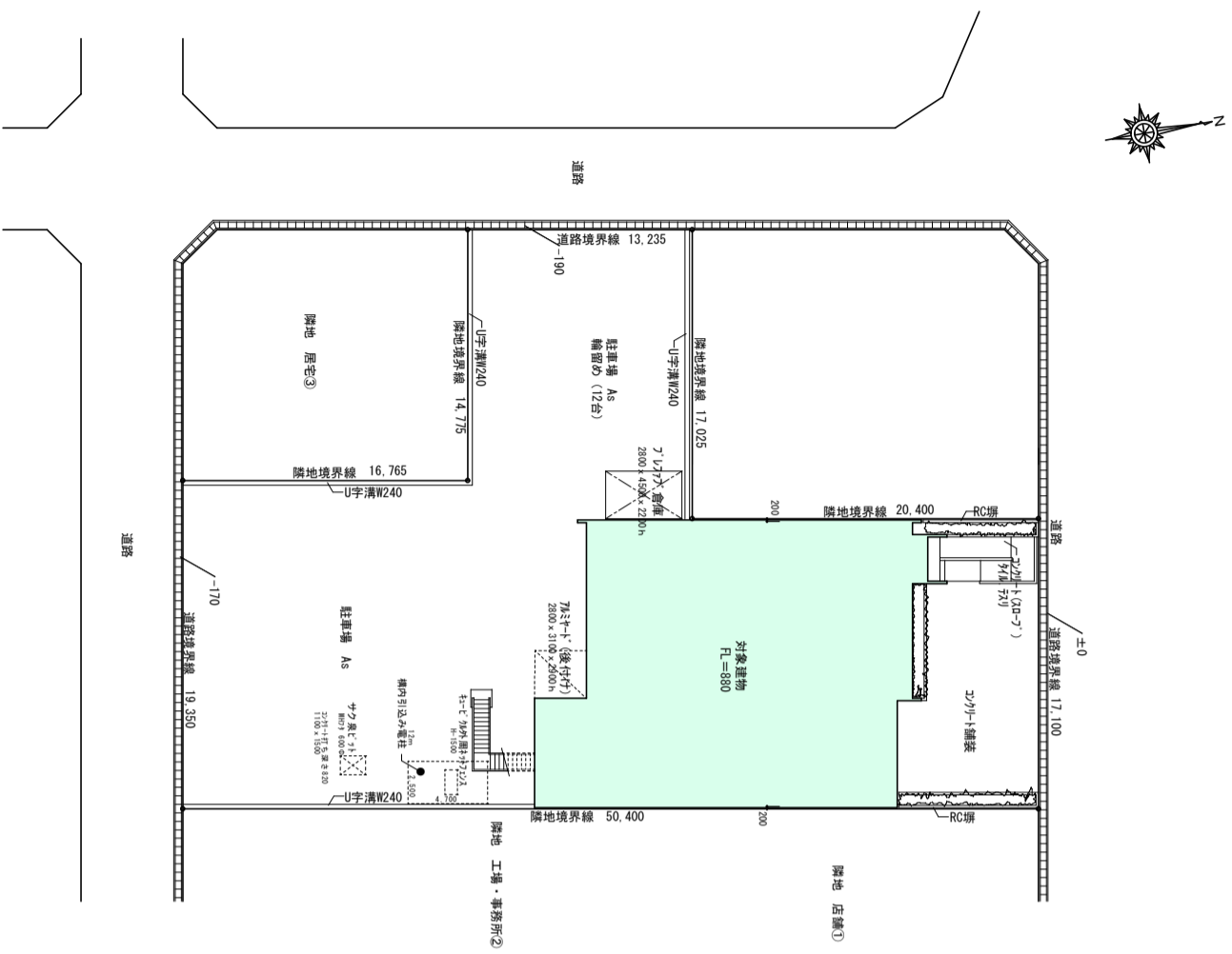
外構図 配置図 1/300
