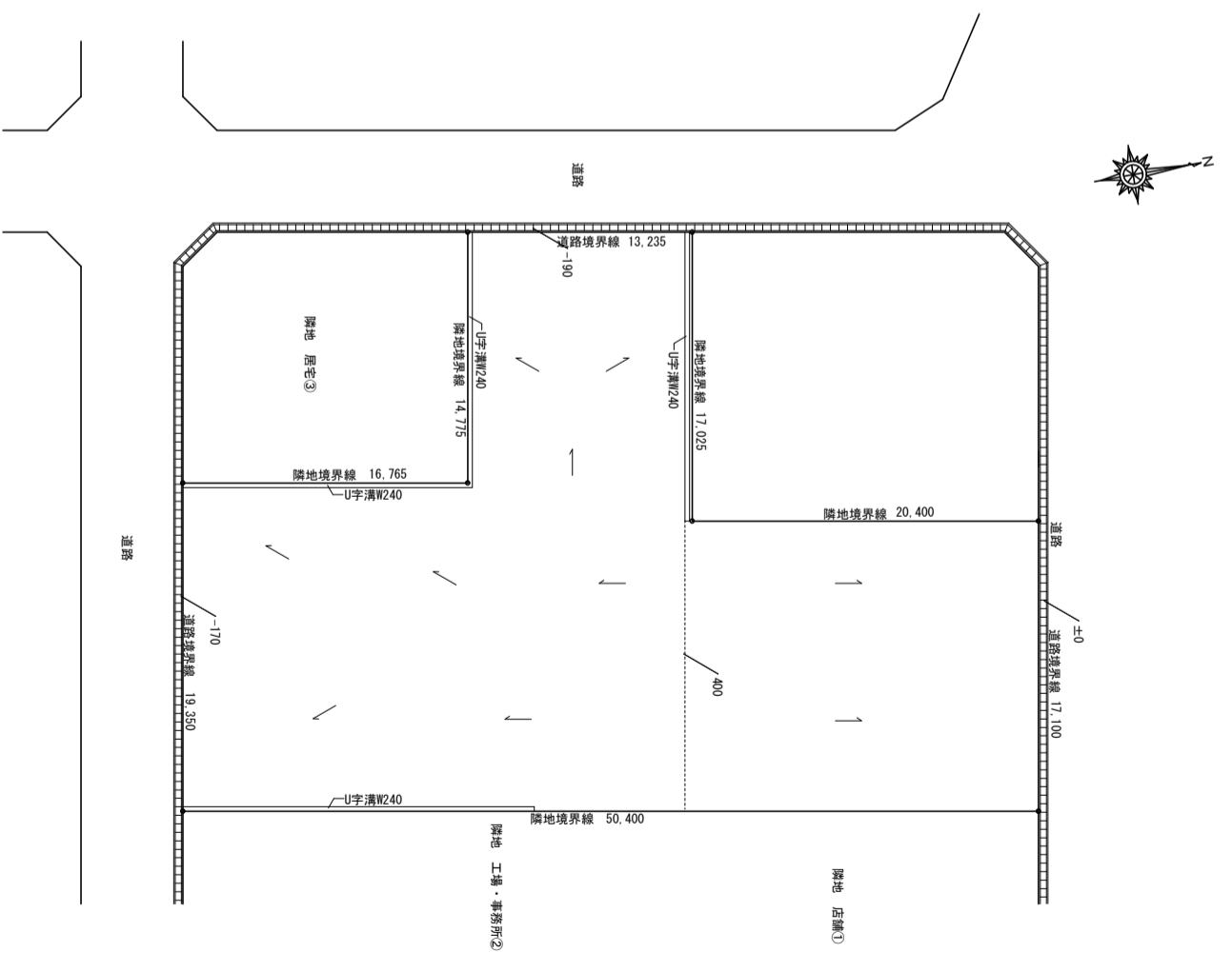
参考図 整地計画レベル図 1/300
