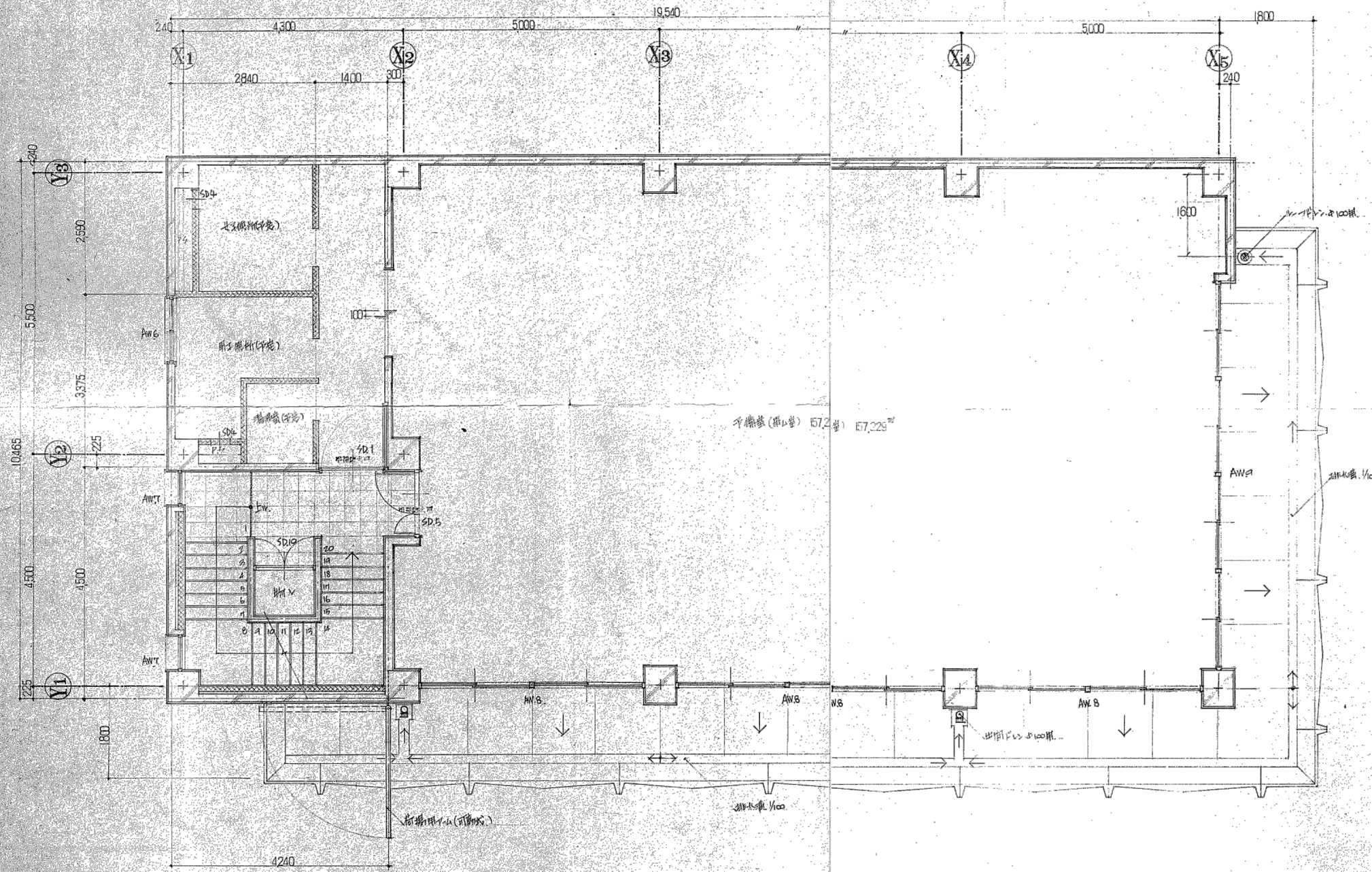
4階平面図 1/50
