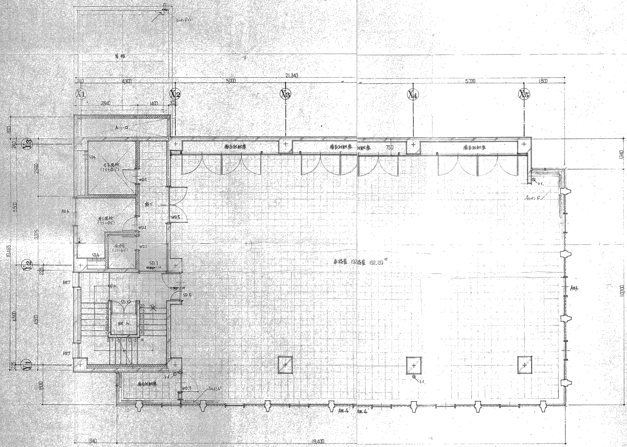
3階平面図 1/50
