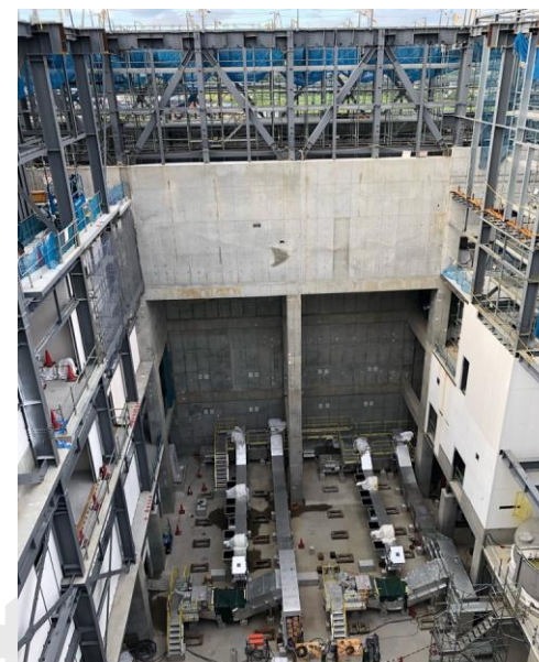
炉室の様子
