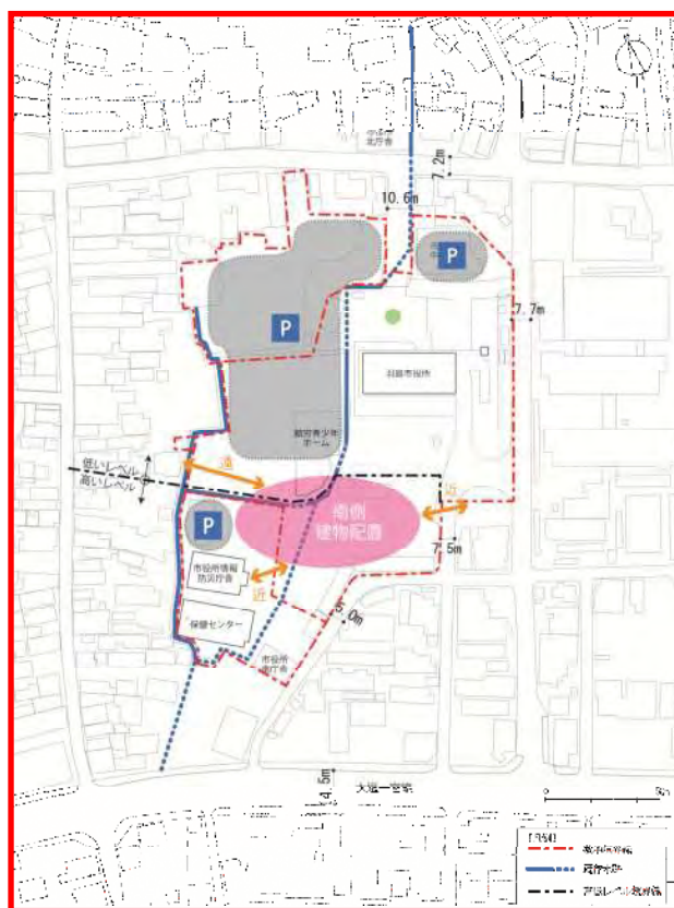
南側配置計画検討図
