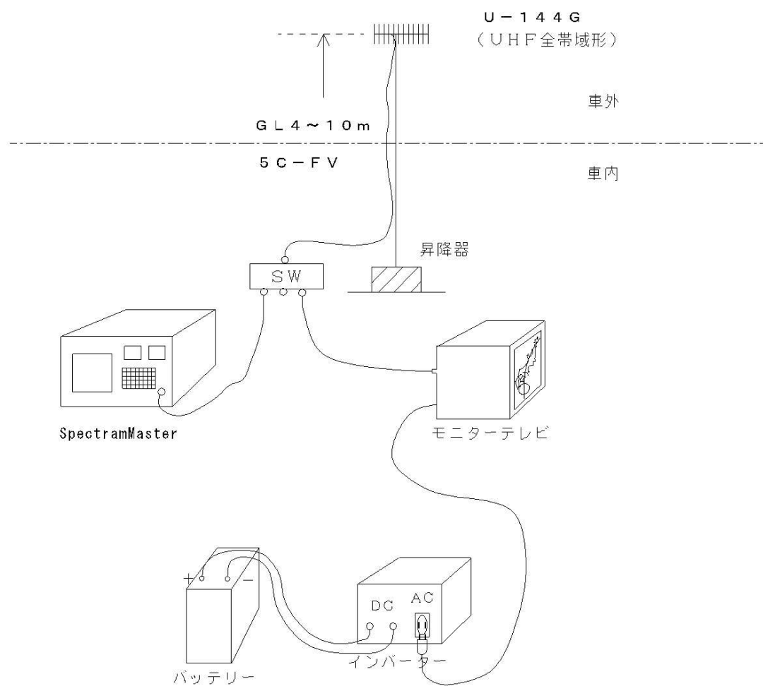
図 8.10-2 電波測定車の概要(アンテナ高さ10m)
